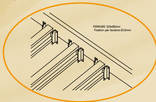
Solution Poutre Industrielle Poutre Kerto/Nail-Web
