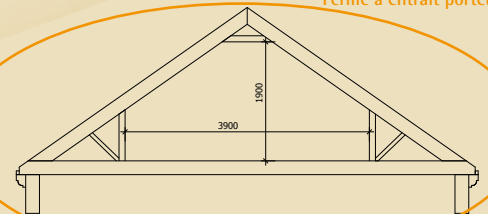
Solution Charpente Industrielle Ferme à entrain porteur
