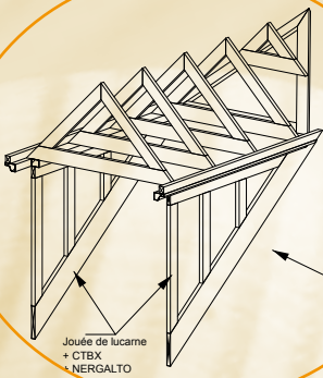
Détail lucarne bois
