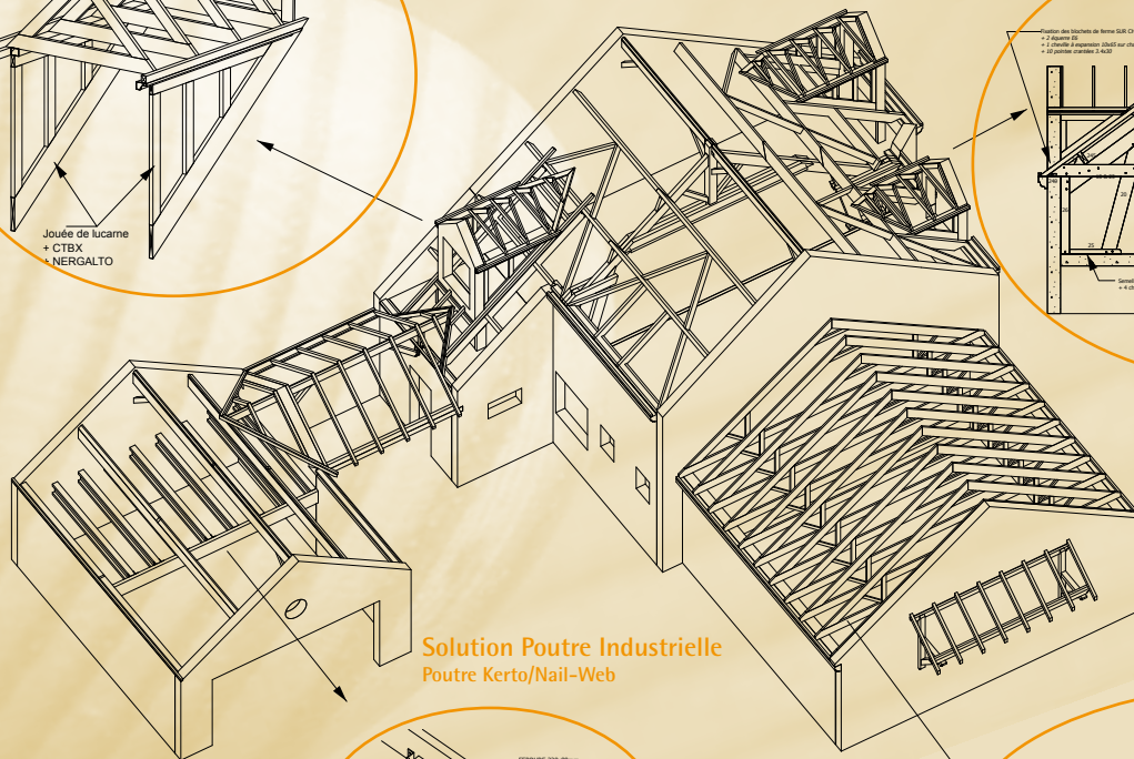
Détail lucarne bois
