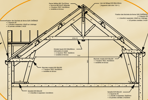
Solution Charpente traditionnelle Ferme traditionnelle sur blochets
